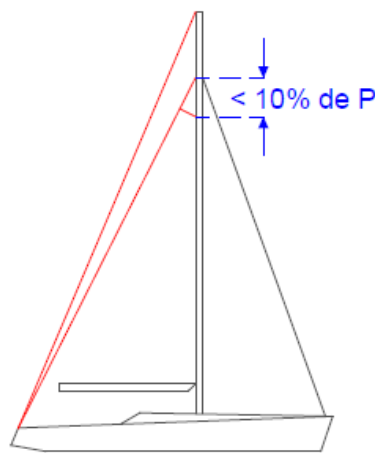
2 ETAIS/GROUPES D'ETAI
